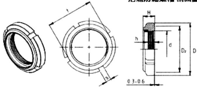
尼龍防鬆螺帽 剖面圖
